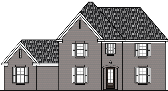
Elevation A
